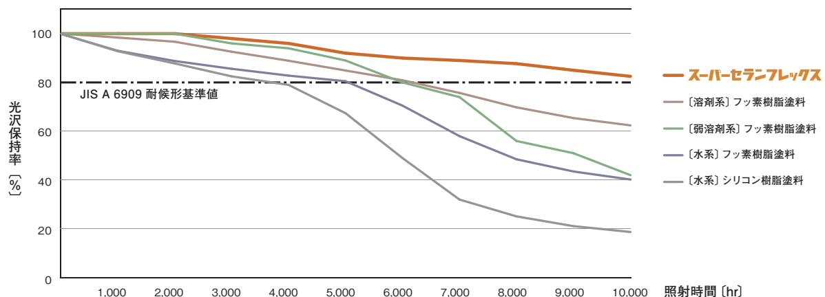
キセノンウェザーメーター 促進耐候性試験
